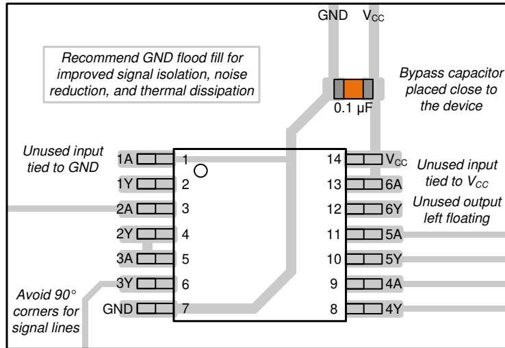
图 11-1. SN74LV6T14-Q1 的示例布局
