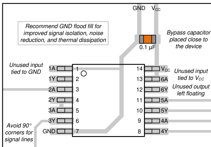
图 11-1. SN74LV6T14 的示例布局
