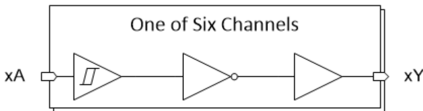
简化逻辑图 (正逻辑)
