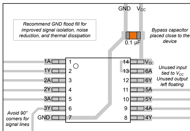
图 9-3. SN74LV6T07-Q1 的示例布局
