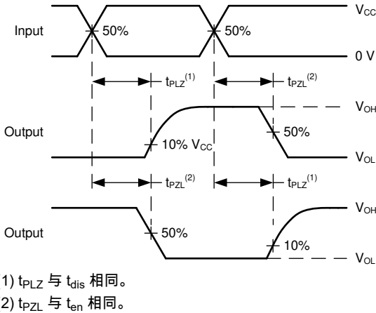
图 7-2. 电压波形传播延迟
