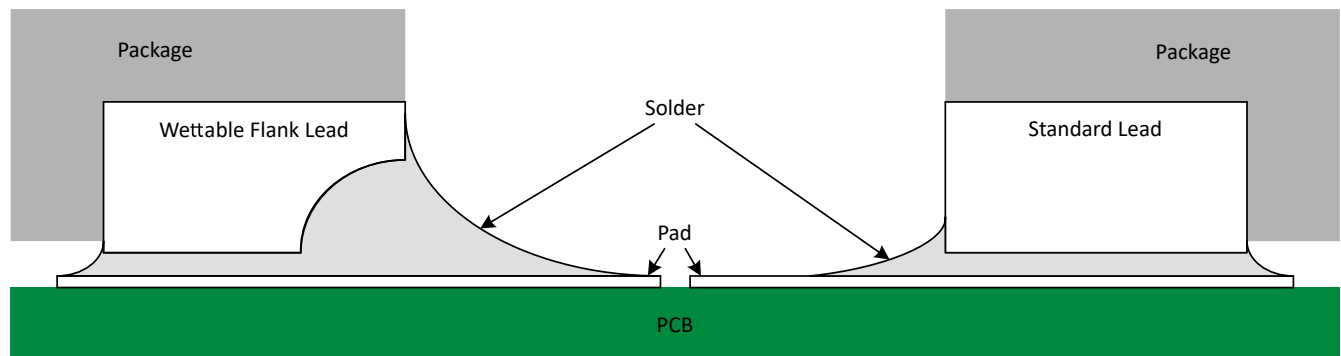
图 8-2. 焊接后具有可润湿侧翼的 QFN 封装和标准 QFN 封装的简化剖面图
