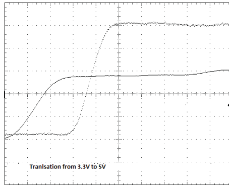
图 8-2. 升压转换
