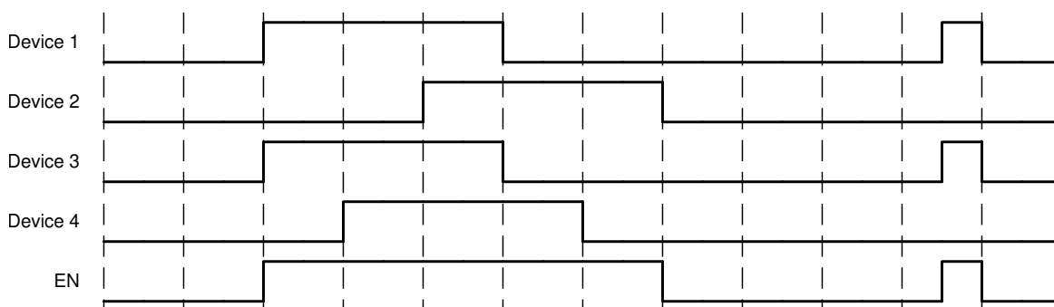
图 9-2. 应用时序图
