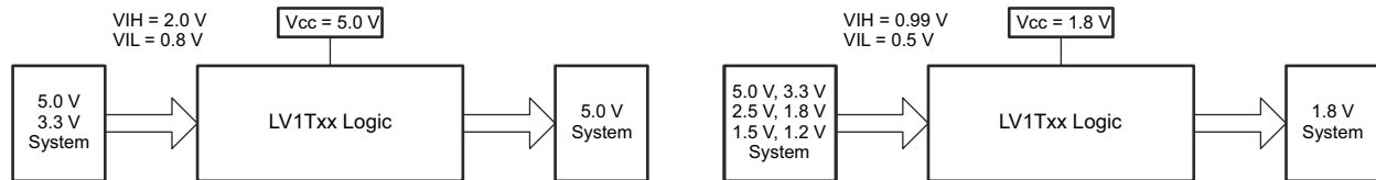
图 8-3. LVxT 升压和降压转换示例
