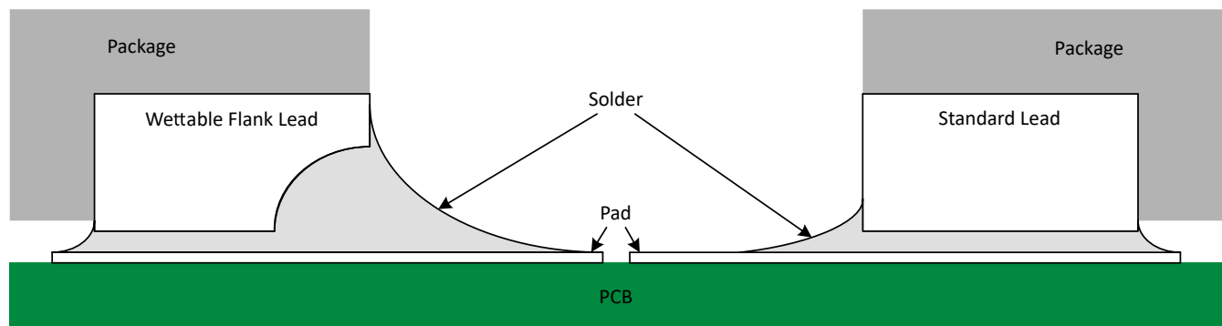
图 8-4. 焊接后具有可润湿侧翼的 QFN 封装和标准 QFN 封装的简化剖面图
