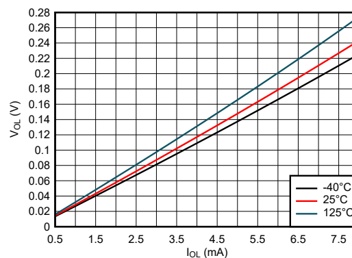
图 6-12. 低电平状态下输出电压与电流间的关系 (1.8V 电源)
