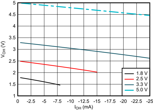
图 6-3. 高电平状态下输出电压与电流间的关系
