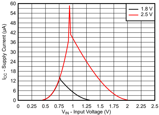
图 6-1. 输入电压范围内的电源电流, 1.8V 和 2.5V 电源
