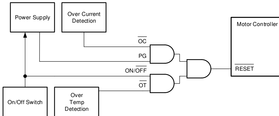
图 10-1. 典型应用框图
