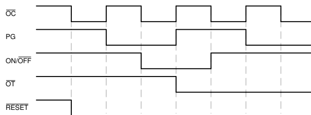
图 10-2. 应用时序图
