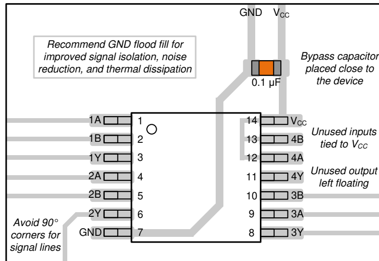
图 12-1. 示例布局 SN74LV4T08-Q1
