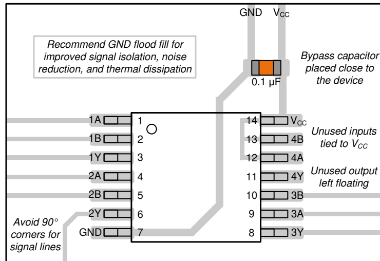
图 10-1. 示例布局 SN74LV4T08-EP
