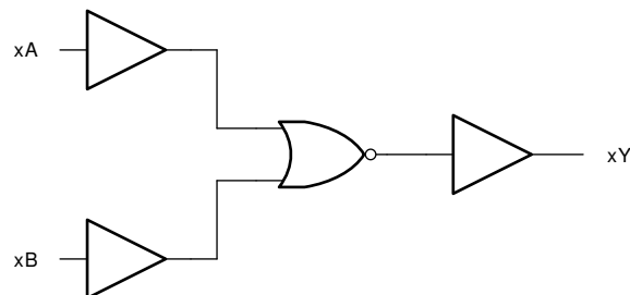
简化逻辑图
