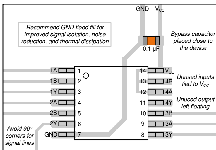
图 12-1. SN74LV4T00-Q1 的示例布局
