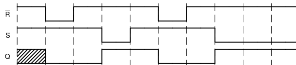
图 10-2. 应用时序图
