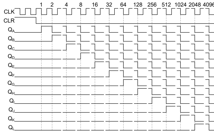
图 9-2. 逻辑时序图
