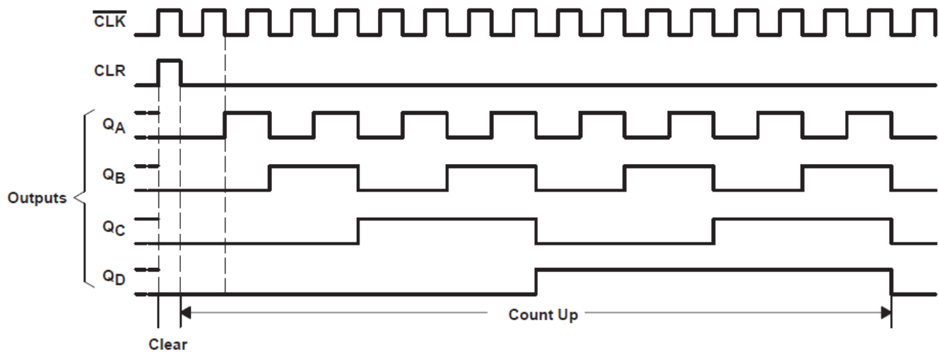
图 6-1. Timing Diagram
