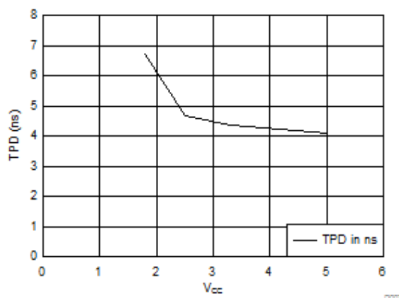
图 5-2. TPD vs V_{CC} at 25^\circ\text{C}
