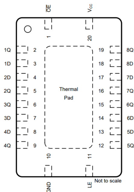
图 4-2. RGY Package 20-Pin VQFN Top View
