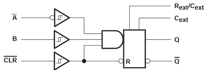
图 6-1. 每个多谐振荡器的逻辑图 (正逻辑)
