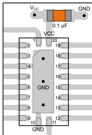
图 7-10. WQFN 和类似封装的旁路电容器放置示例
