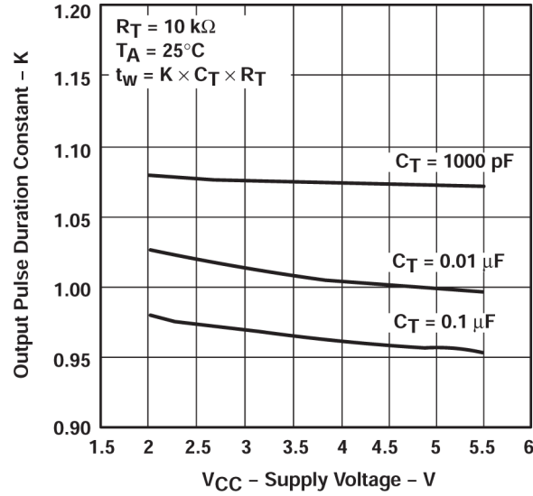
图 7-6. 输出脉冲持续时间常数与电源电压的关系
