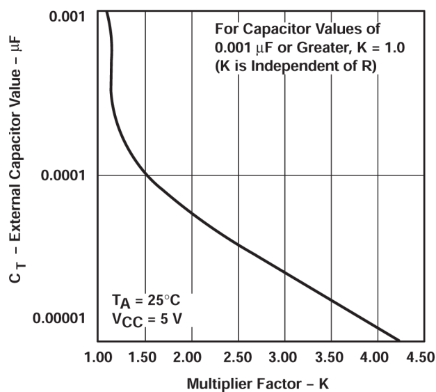
图 7-5. 外部电容与倍乘因子之间的关系
