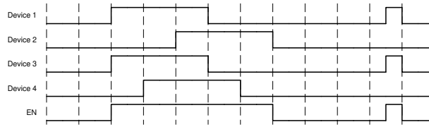
图 8-2. 应用时序图
