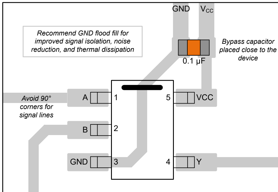
图 8-3. SN74LV1T32-Q1 的示例布局
