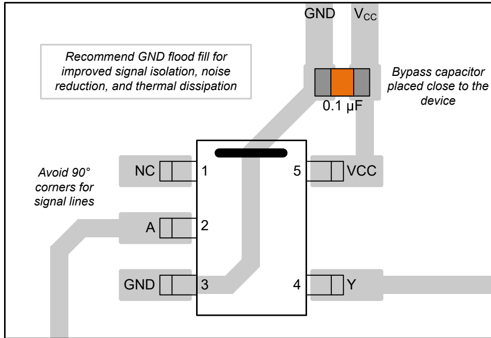
图 10-1. SN74LV1T04-Q1 的示例布局
