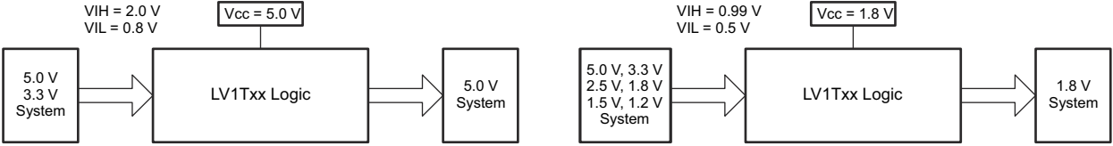
图 7-2. LVxT 升压和降压转换示例
