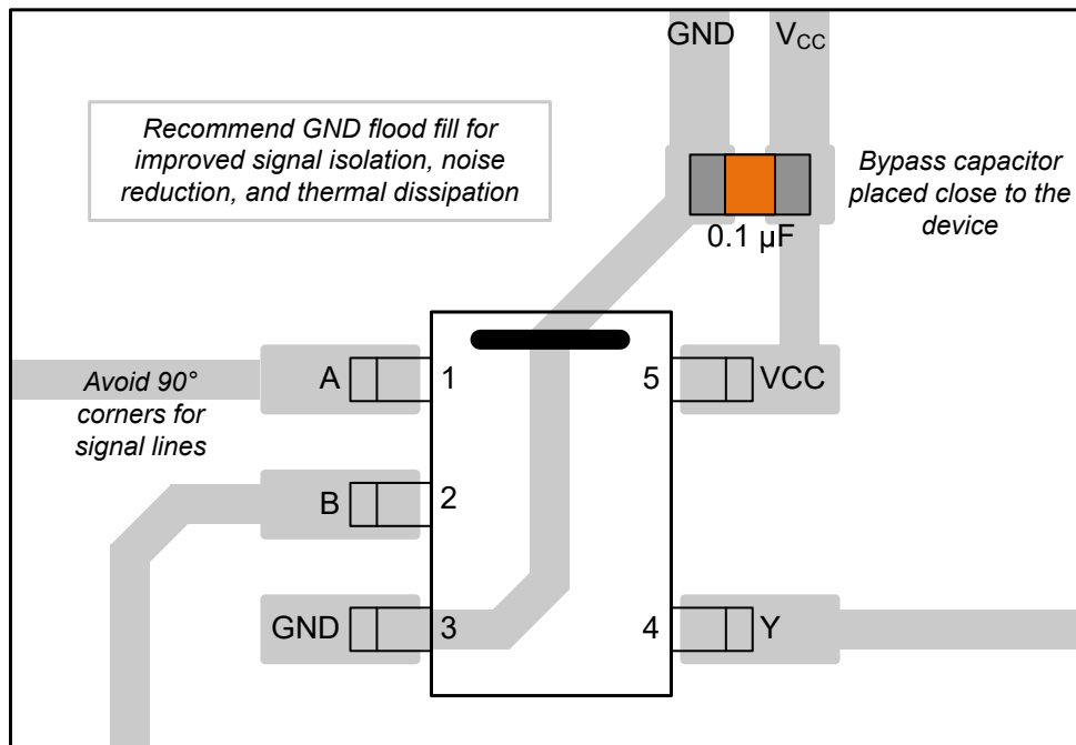
图 8-3. SN74LV1T00-Q1 的示例布局
