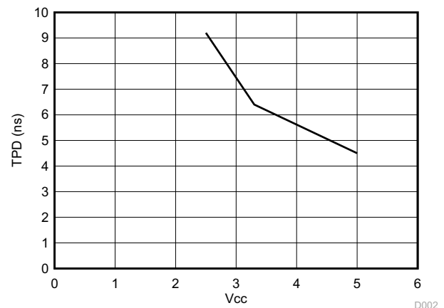
图 6-3. TPD vs. V CC at 25°C
