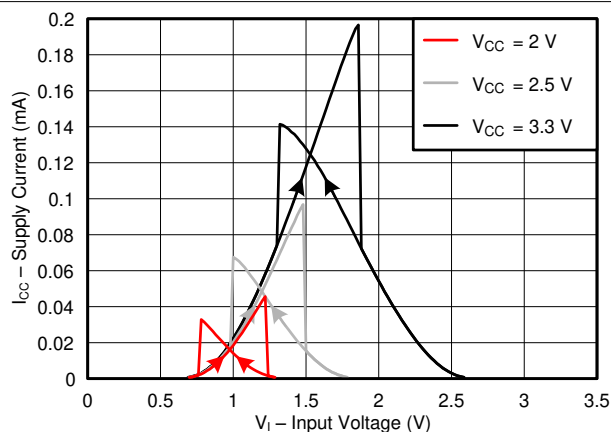
图 6-3. 2V、2.5V 和 3.3V 输入电压电源上的电源电流
