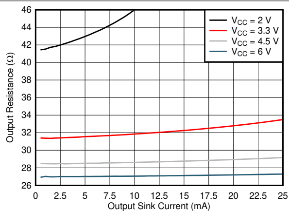
图 6-1. 低电平状态下的输出驱动器电阻
