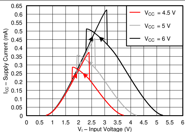
图 6-4. 4.5V、5V 和 6V 输入电压电源上的电源电流
