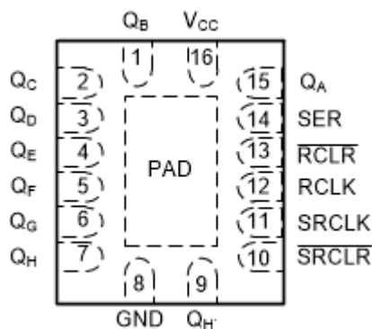
BQB 或 WBQB 封装， 16 引脚 WQFN (顶视图)
