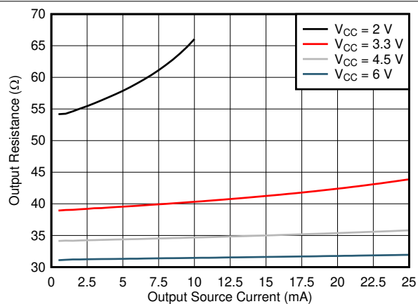
图 6-2. 高电平状态下的输出驱动器电阻
