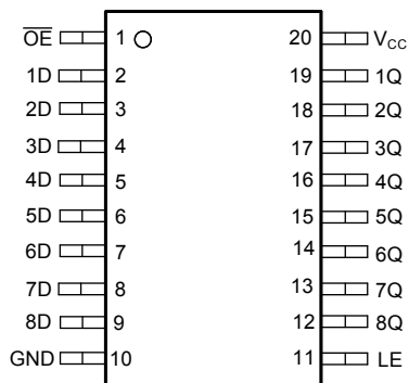
图 5-1. DGS Package 20-Pin VSSOP Top View
