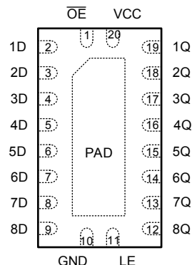
图 5-2. RKS Package 20-Pin VQFN Top View
