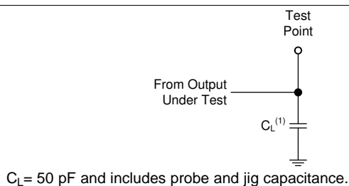
图 5. Load Circuit
