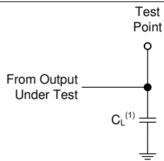
图 5. Load Circuit
