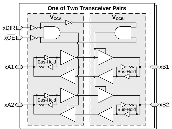
功能方框图
