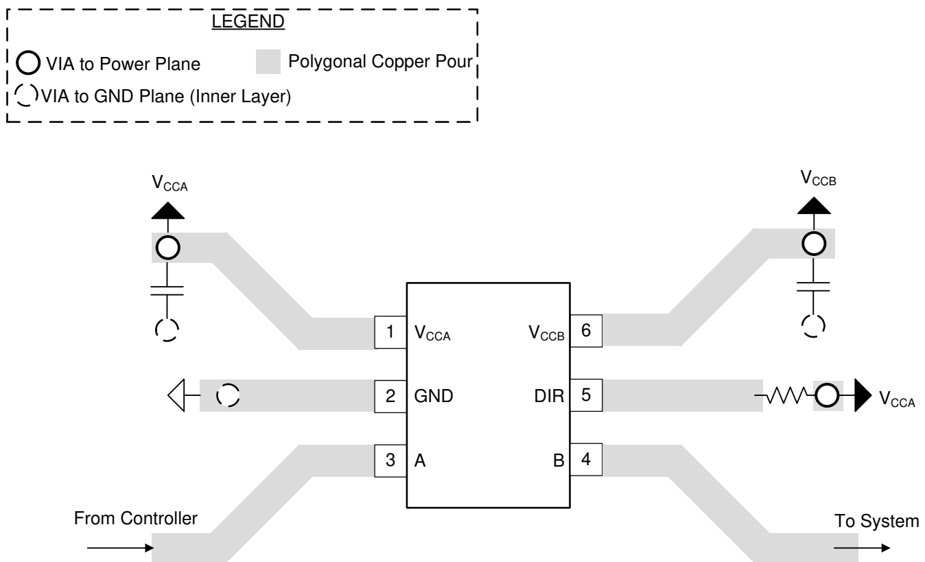
图 11-1. PCB Layout Example
