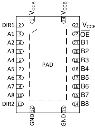
图 4-2. RHL 和 WRGY 封装, 24 引脚 VQFN (俯视图)
