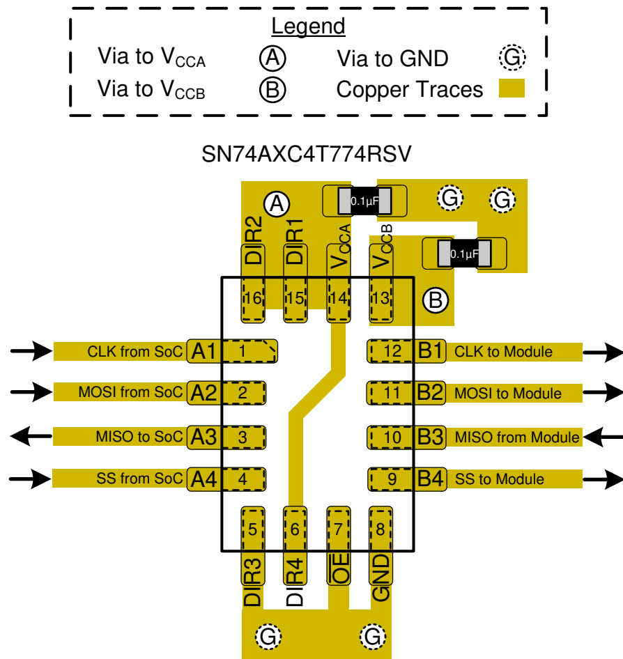
图 8-3. 布局示例
