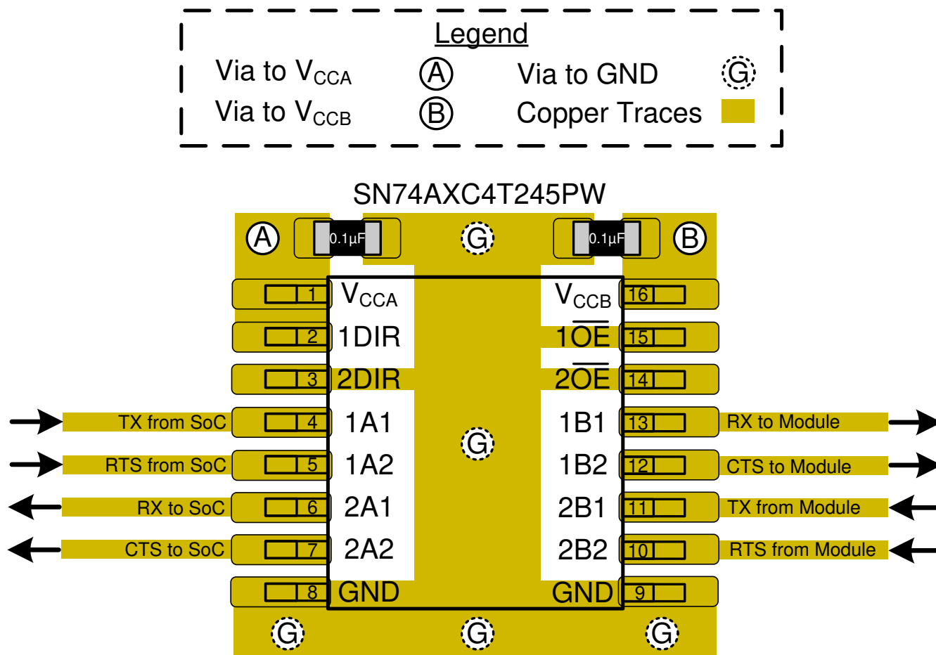
图 8-3. 布局示例
