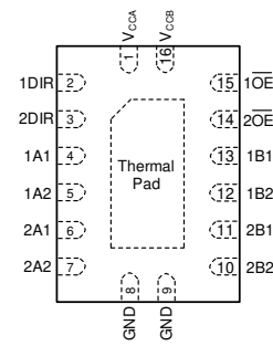
图 4-2. BQB 封装 16 引脚 WQFN（透明顶视图）
