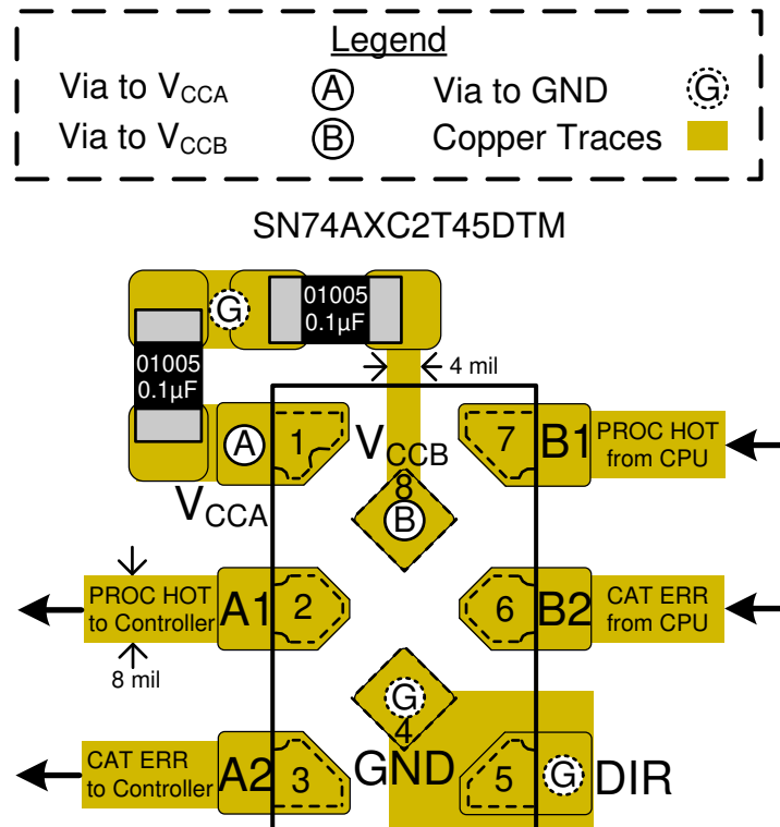
图 8-3. SN74AXC2T45DTM 布局示例
