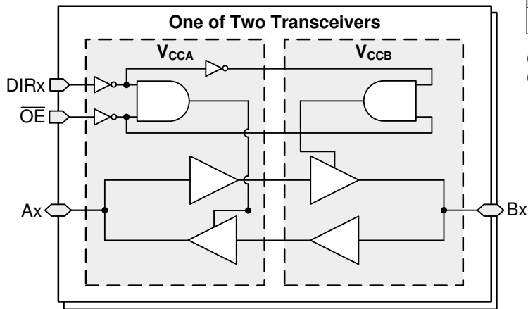
功能方框图
