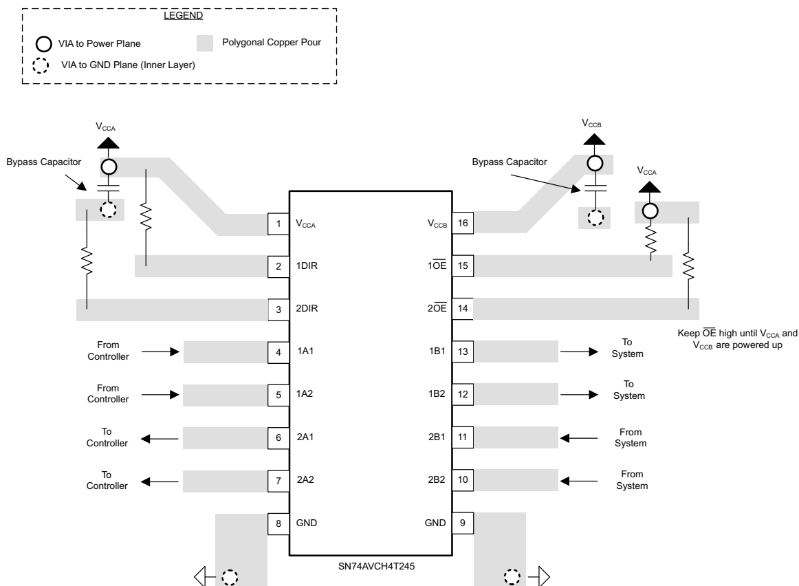
图 8-3. Layout Recommendation
