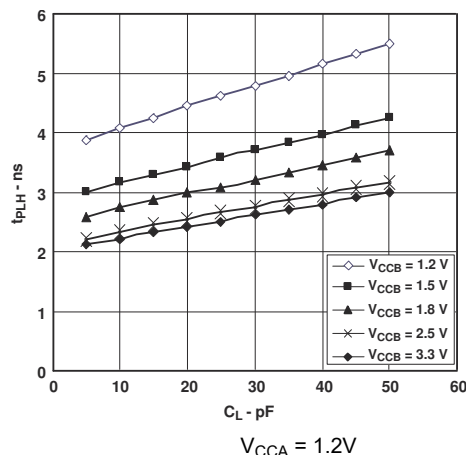
图 6-2. 典型传播延迟 (A 至 B) 与负载电容间的关系
