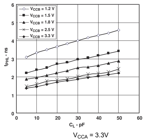
图 6-10. 典型传播延迟 (A 至 B) 与负载电容间的关系
