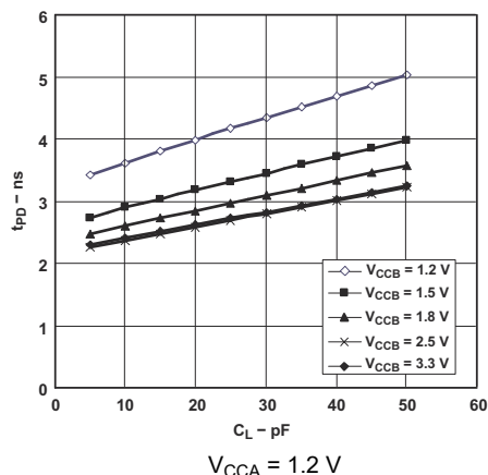
图 5-1. 典型传播延迟 (A 至 B) 与负载电容间的关系
