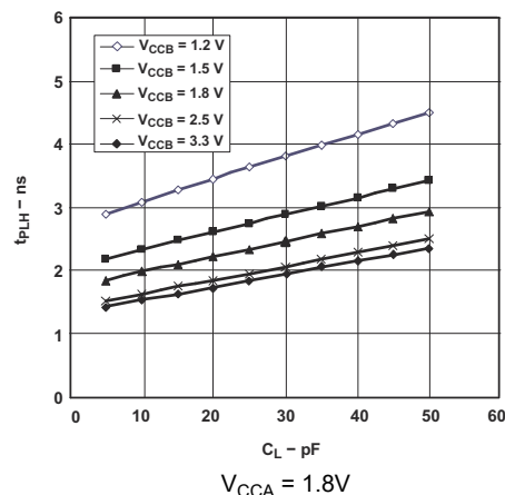
图 5-4. 典型传播延迟 (A 至 B) 与负载电容间的关系
