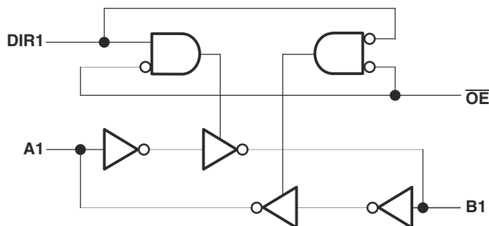
图 7-1. SN74AVC4T774-Q1 逻辑图 (正逻辑)
