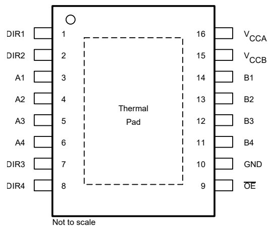
图 4-2. DYY 封装，16 引脚 SOT (顶视图)
