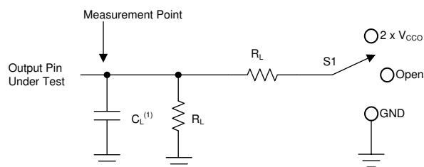
图 6-1. Load Circuit
