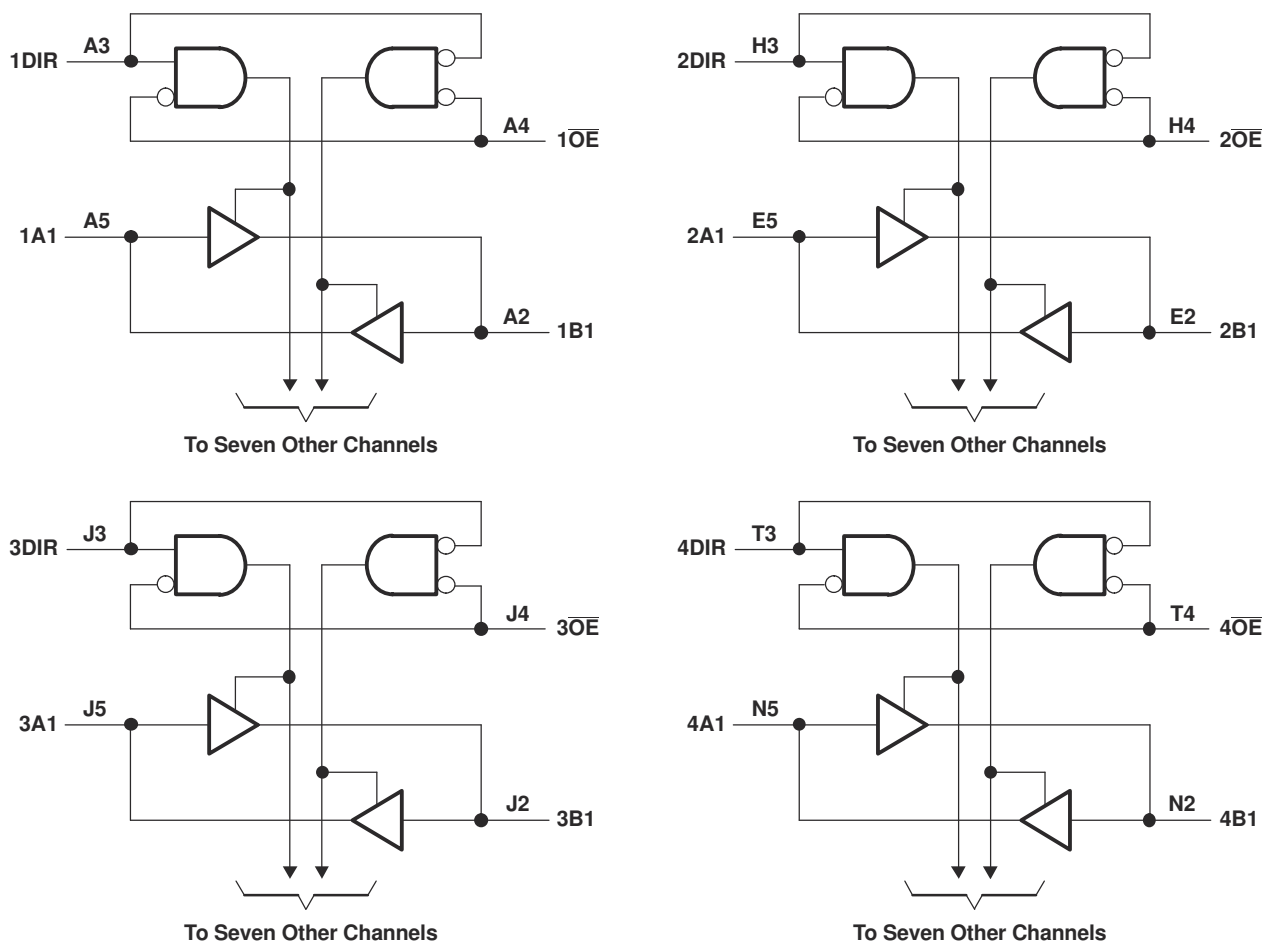
逻辑图 (正逻辑)
