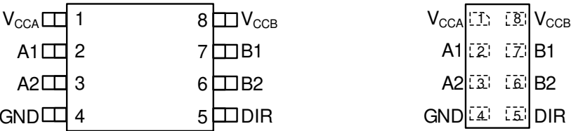
图 4-1. DCU ( 8 引脚 VSSOP ) 和 DTT ( 8 引脚 SON ) 封装 ( 顶视图 )
