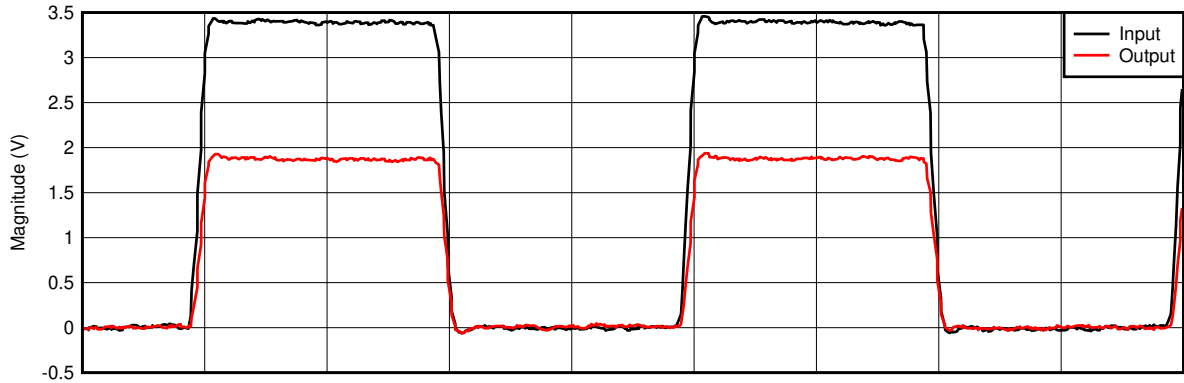
图 8-2. 利用 1MHz 方波实现 3.3V 至 1.8V 电平转换
