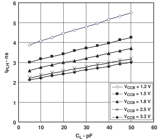
图 5-2. 低电平到高电平 (B 到 A) 的典型传播延迟与负载电容间的关系 T_A = 25^\circ\text{C} , V_{CCA} = 1.2\text{V}
