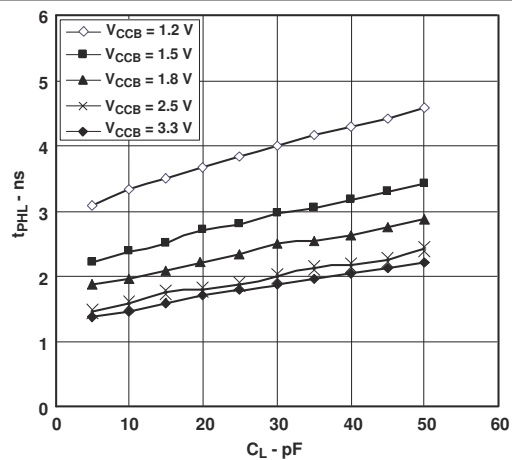
图 5-10. 低电平到高电平 (B 到 A) 的典型传播延迟与负载电容间的关系 T_A = 25^\circ\text{C} , V_{CCA} = 3.3V
