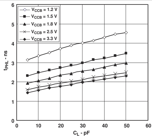
图 5-8. 低电平到高电平 (B 到 A) 的典型传播延迟与负载电容间的关系 T_A = 25^\circ\text{C} , V_{CCA} = 2.5V
