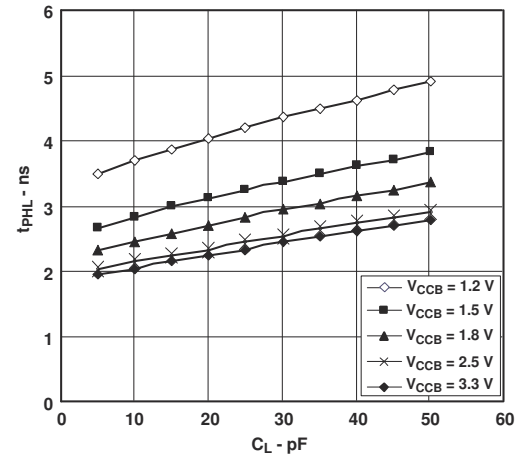
图 5-4. 低电平到高电平 (B 到 A) 的典型传播延迟与负载电容间的关系 T_A = 25^\circ\text{C} , V_{CCA} = 1.5\text{V}
