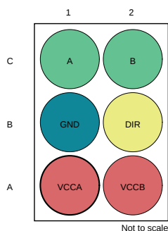
图 4-4. YZP 封装， 6 引脚 DSBGA ( 底视图 )
