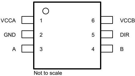
图 4-3. DRL 封装，6 引脚 SOT-5X3 ( 顶视图 )
