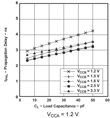
图 6-2. 典型传播延迟 t_{PHL} (A 到 B) 与负载电容间的关系
