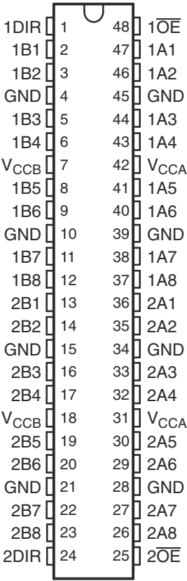
图 5-1. DGV 封装 48 引脚 TVSOP 顶视图
