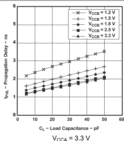
图 6-10. 典型传播延迟 t_{PHL} (A 到 B) 与负载电容间的关系
