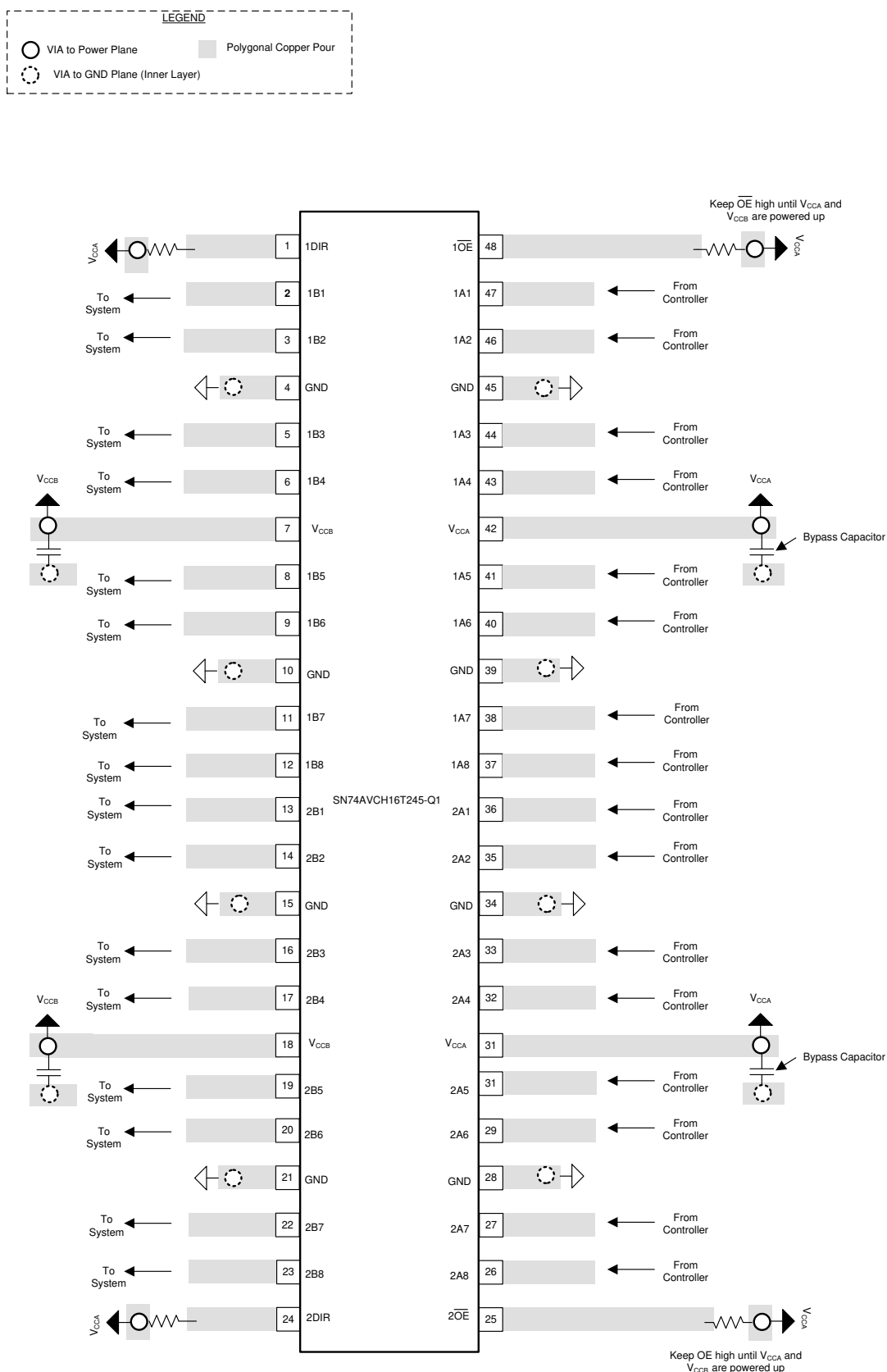
图 11-1. 推荐布局示例
