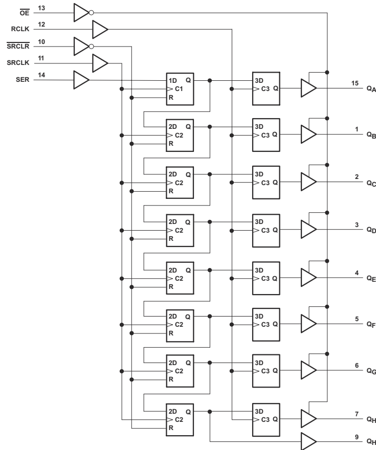
简化原理图
