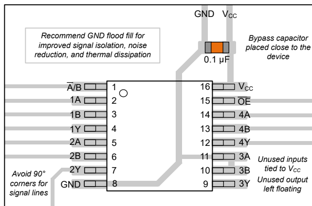
图 8-3. SN74AHCT257 的示例布局
