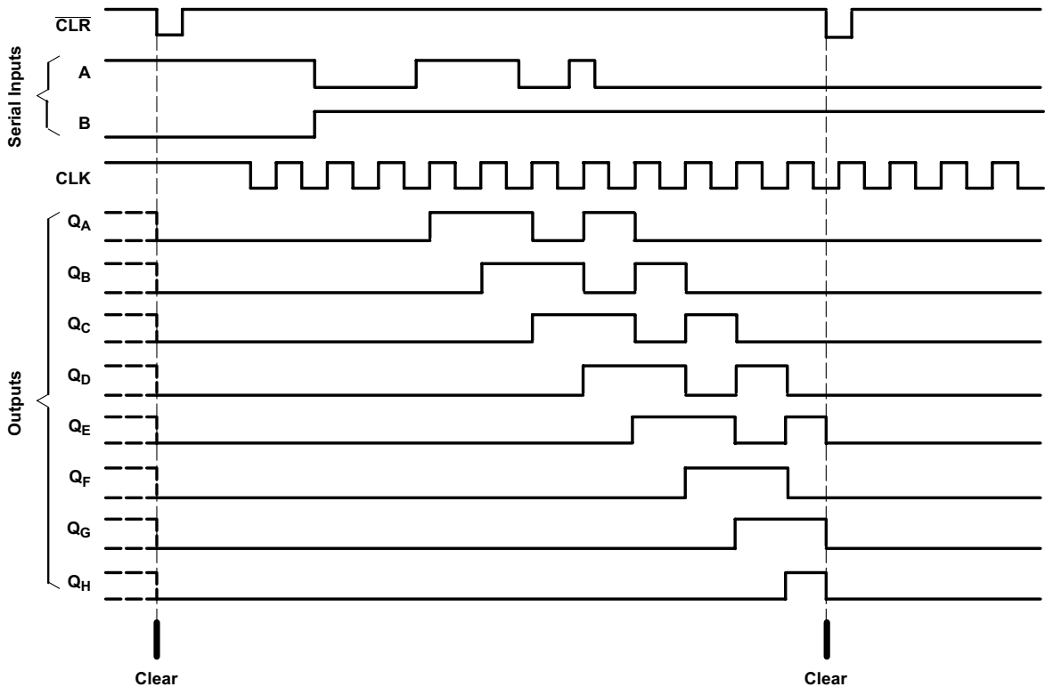
图 8-2. 应用时序图
