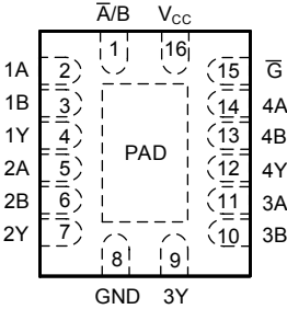
图 4-2. WBQB 封装，16 引脚 WQFN（透明顶视图）
