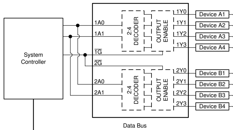
图 8-1. 典型应用框图
