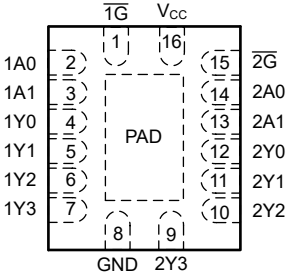
图 4-2. BQB 封装， 16 引脚 WQFN (顶视图)
