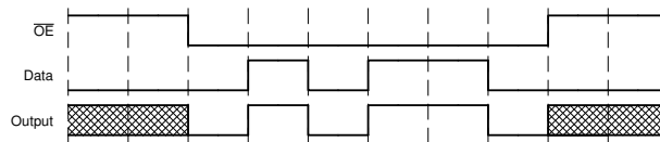
图 9-2. 应用时序图
