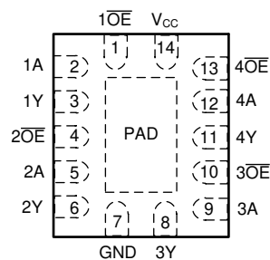
图 5-2. BQA 封装，14 引脚 WQFN ( 顶视图 )
