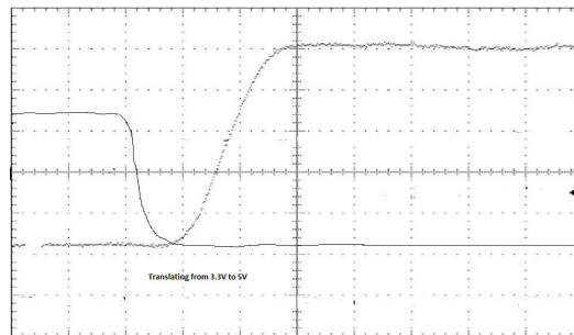
图 8-3. Up Translation
