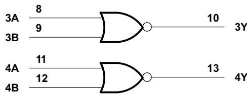
逻辑图 (正逻辑)
