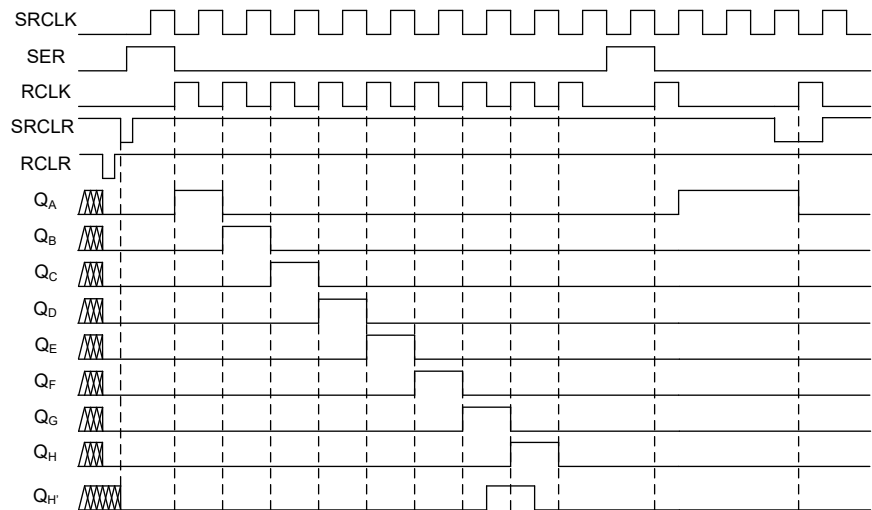
图 5-1. 时序图
